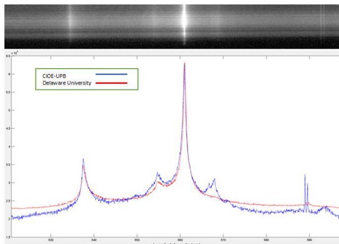
Figura 20. Fotografía del espectro del Pb vista por la cámara CCD y comparación de espectros LIBS obtenidos con el prototipo y un espectro patrón.
