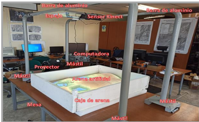
Figura 4. Prototipo GS-Sandbox
